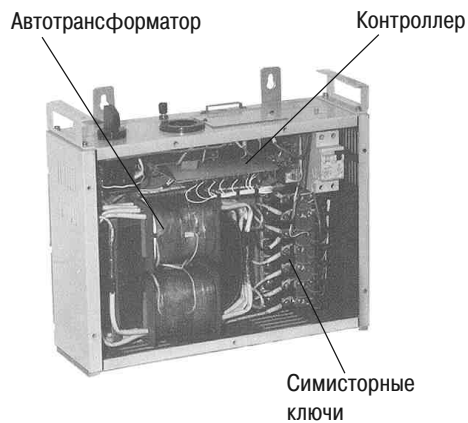
Рис. 8. Устройство стабилизатора
