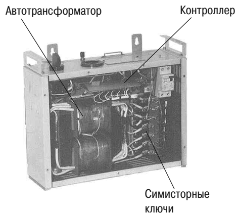
Рис. 8. Устройство стабилизатора
