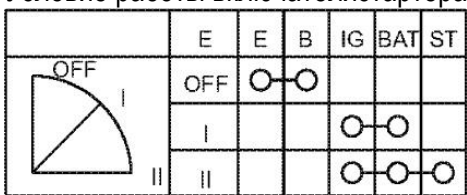
Условие работы включателя стартера
