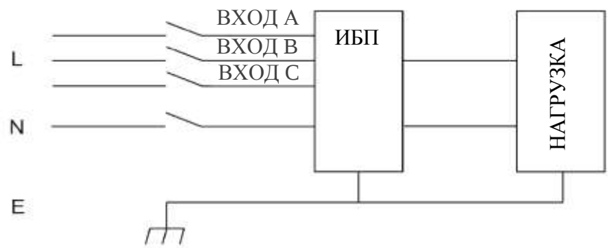
Рисунок 2.1 – Схема подключения ИБП
