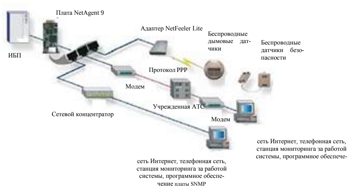
Рисунок 1.6 – Типовая топология сетевого управления ИБП
