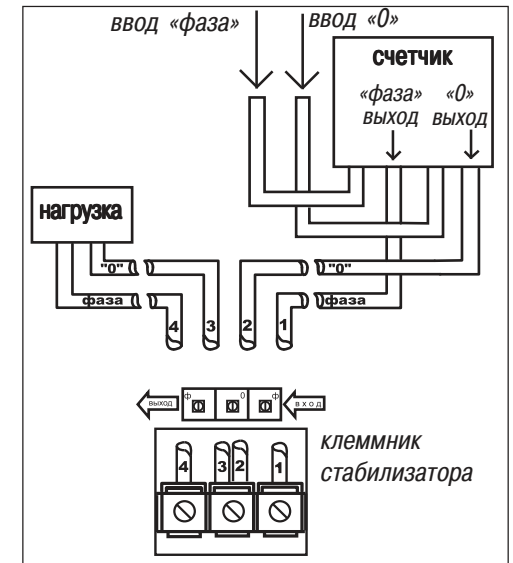
Рис. 17. Схема установки
