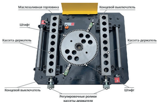
Рис. 3Б Вид с поднятой крышкой GW 42A
