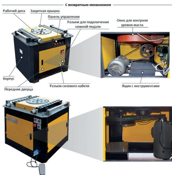
Рис. 1 Общий вид
