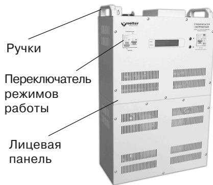
Рис. 1. Стабилизатор напряжения
