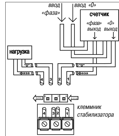
Рис. 17. Схема установки
