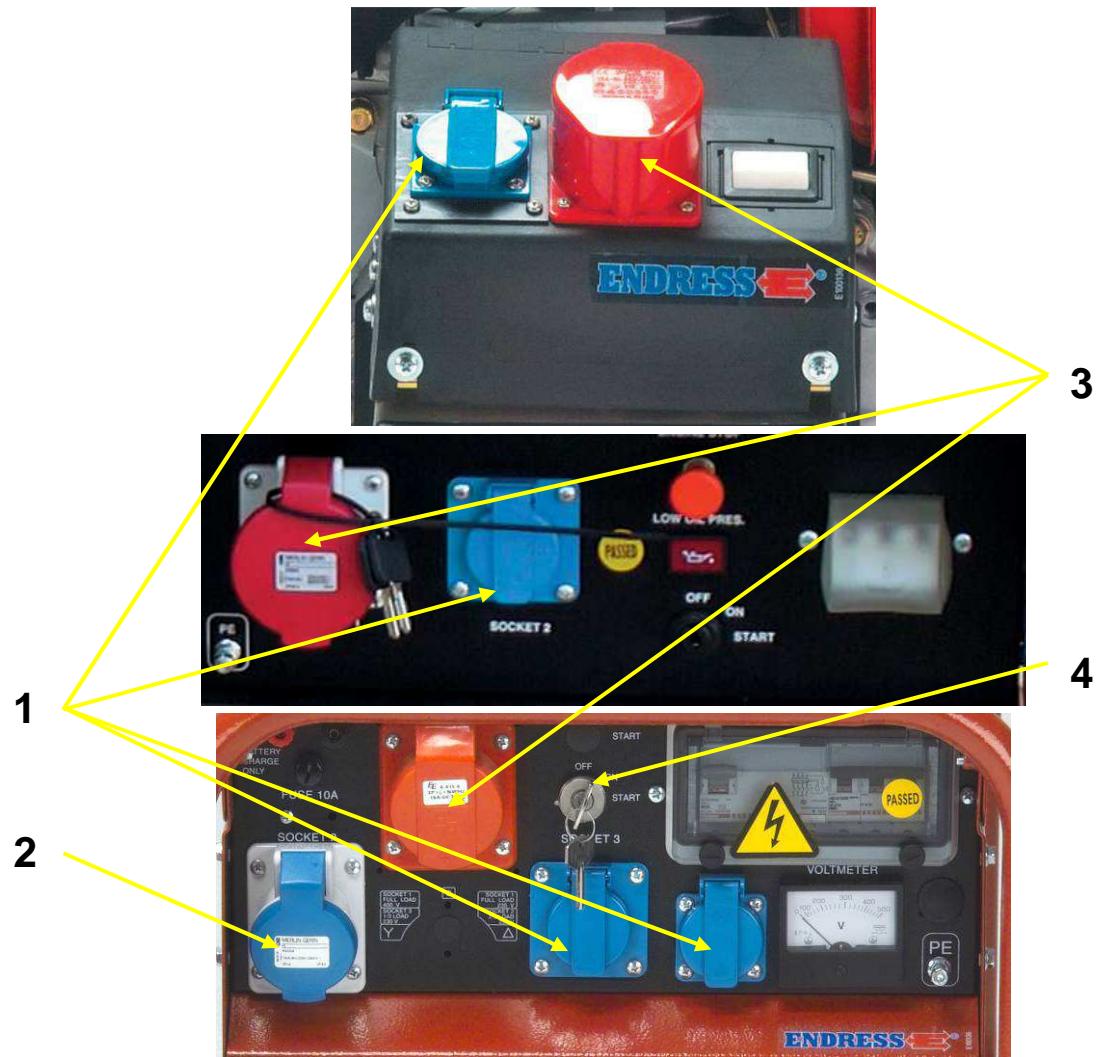
Рис. 4.4: Подключение потребителей
