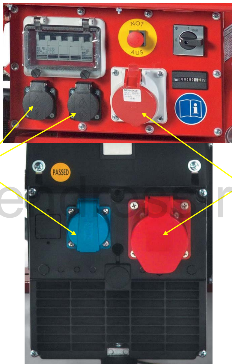
Рис. 4.4: Подключение потребителей
