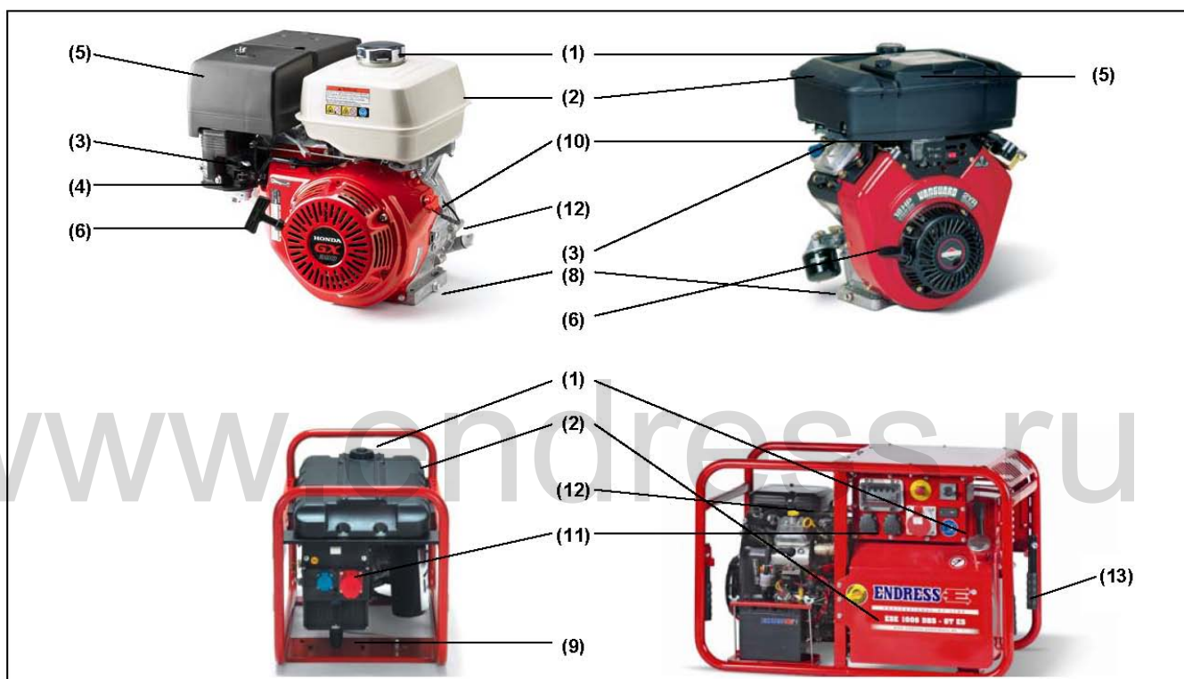
Рис 3.1. Элементы электростанции
