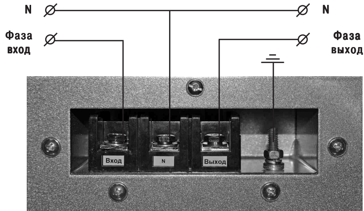
Рис. 2. Схема подключения стабилизатора
