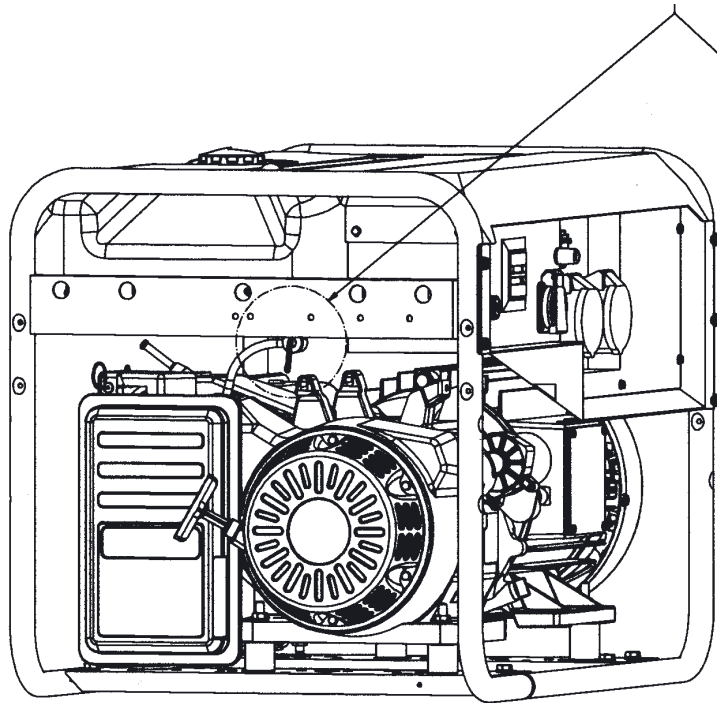
Топливный кран
